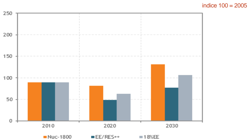
Graphique 30. Evolution des émissions de gaz à effet de serre du parc électrique belge dans les scénarios Nuc-1800 , EE/RES++ et 18%EE
