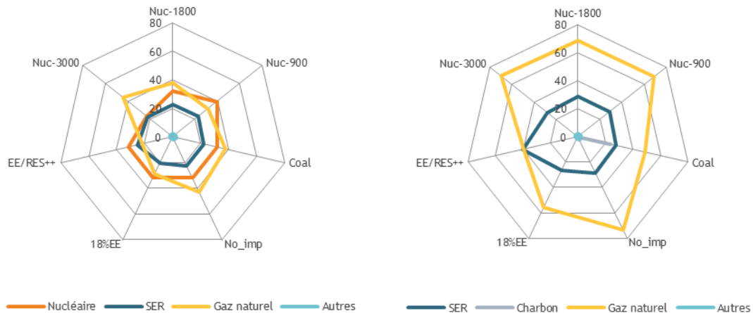
Graphique 33. Production d'électricité par forme d'énergie, 2020 (gauche) et 2030 (droite)
