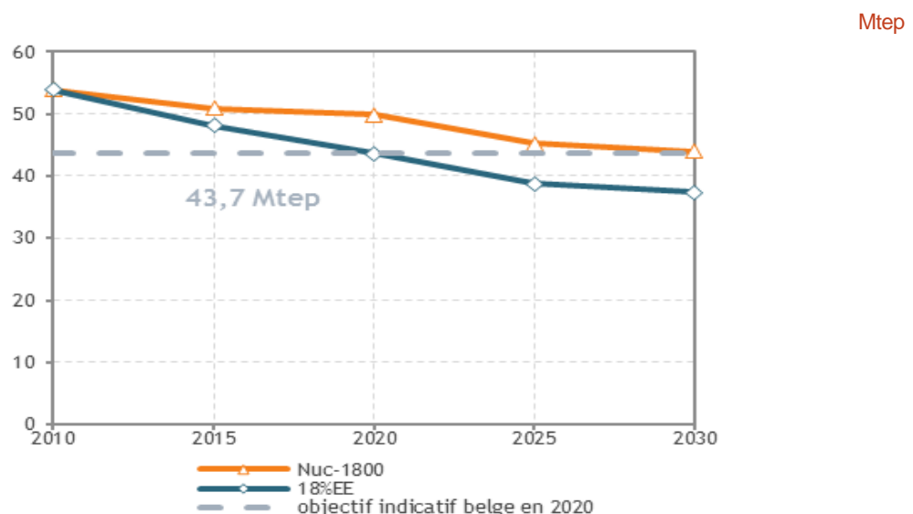
Graphique 18. Evolution de la consommation d'énergie primaire dans les scénarios 18%EE et Nuc-1800 , 2010-2030
