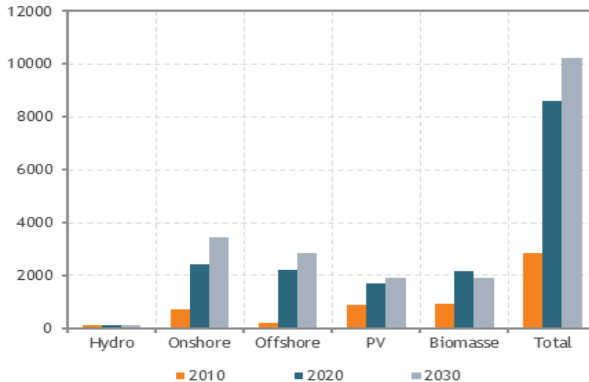
Graphique 9. Evolution de la capacité installée des unités SER, scénario Nuc-1800
