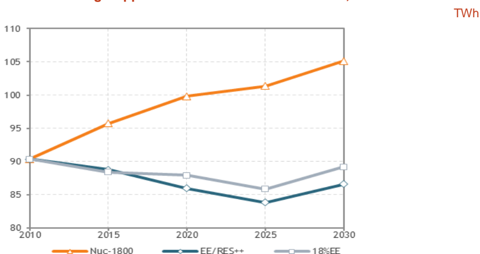
Graphique 26. Evolution de l'énergie appelée dans les scénarios Nuc-1800 , EE/RES++ et 18%EE
