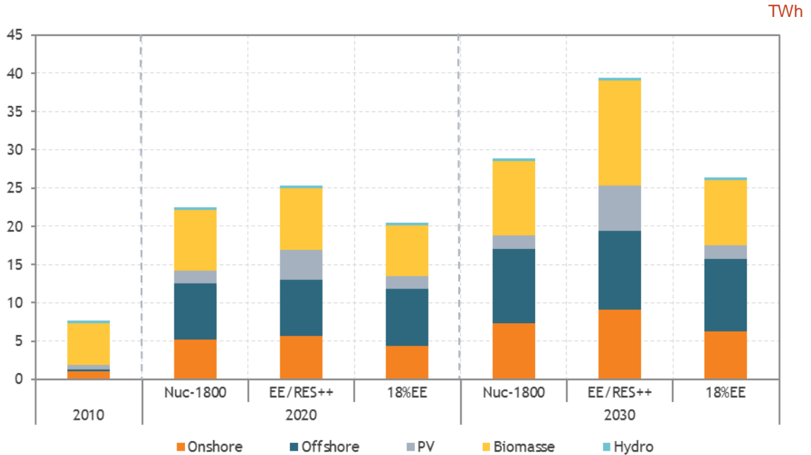
Graphique 28. Evolution de la production d'électricité à partir de SER dans les scénarios Nuc-1800, EE/RES++ et 18%EE
